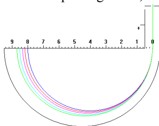
Espectrómetro Brainbridge © Ángel Franco García
